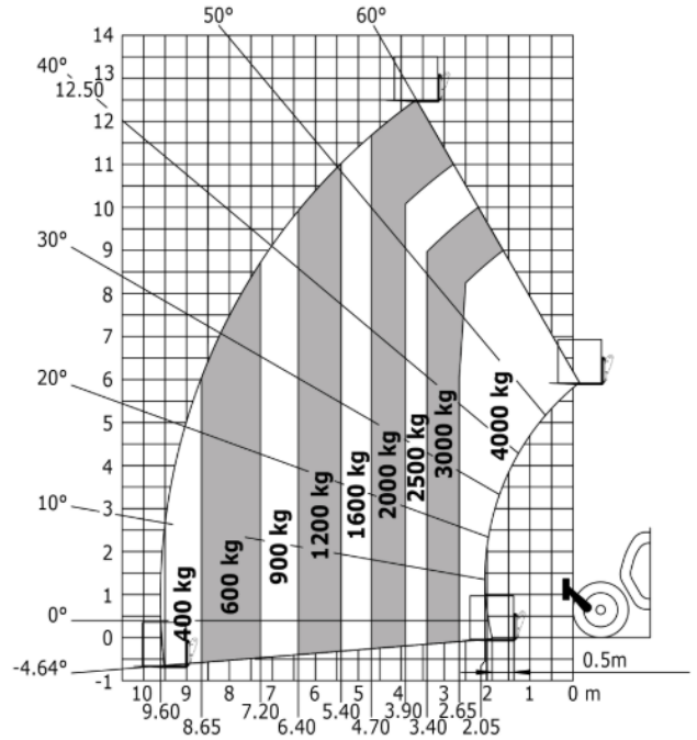
Load chart (EN1459-B) with stabilisers :
